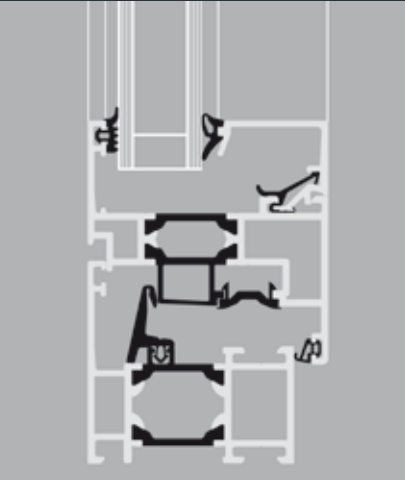
Schüco Novonic, който пести енергия Schüco Novonic mit der Beschlagsnut, die Energie spart
